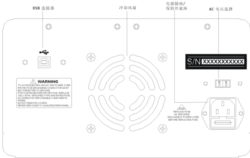
Fig.1.5-1 MPD-3303S/3303D/3305D 后面板图
