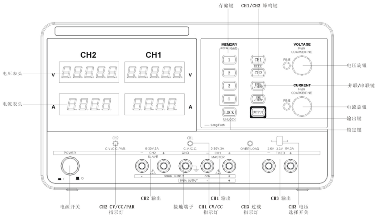
Fig.1.4-1 MPD-3303S 前面板图
